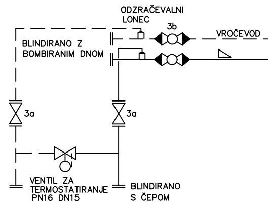
15/3: VGRADNJA TERMOSTATIRANE KRATKE VEZI ZARADI VAROVANJA PRED ZMRZOVANJEM (ZAČASNI ZAKLJUČEK VROČEVODA)
