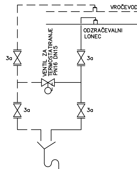
15/4: VGRADNJA TERMOSTATIRANE KRATKE VEZI ZARADI VAROVANJA PRED ZMRZOVANJEM (ODZRAČEVANJE V NEOGREVANEM PROSTORU ALI NA PROSTEM)
