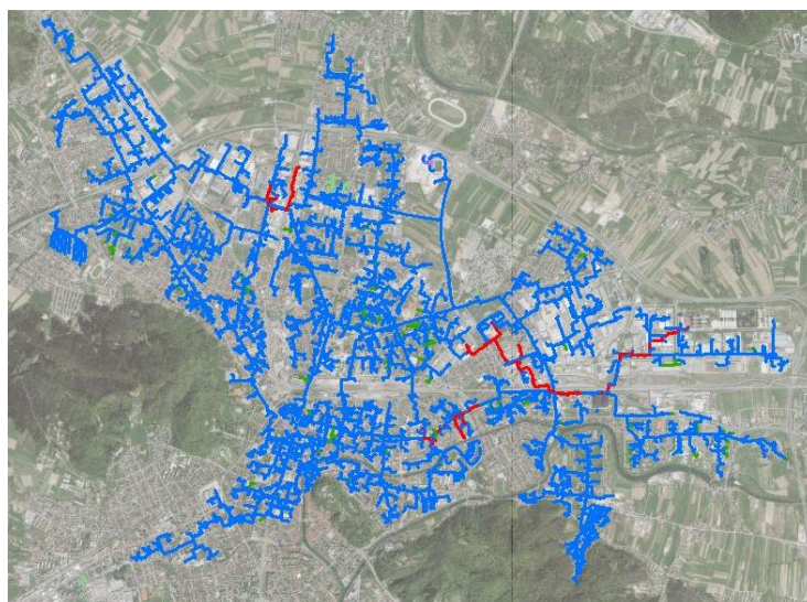
Slika 1: Vročevodno omrežje JPE
